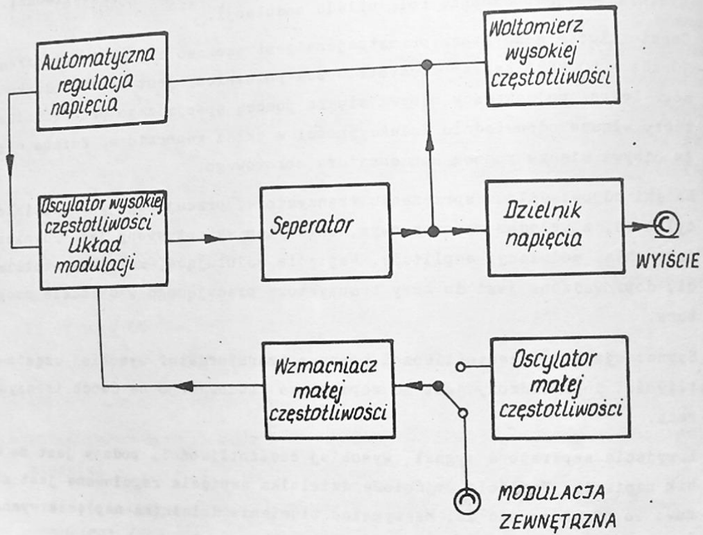
Schemat blokowy
